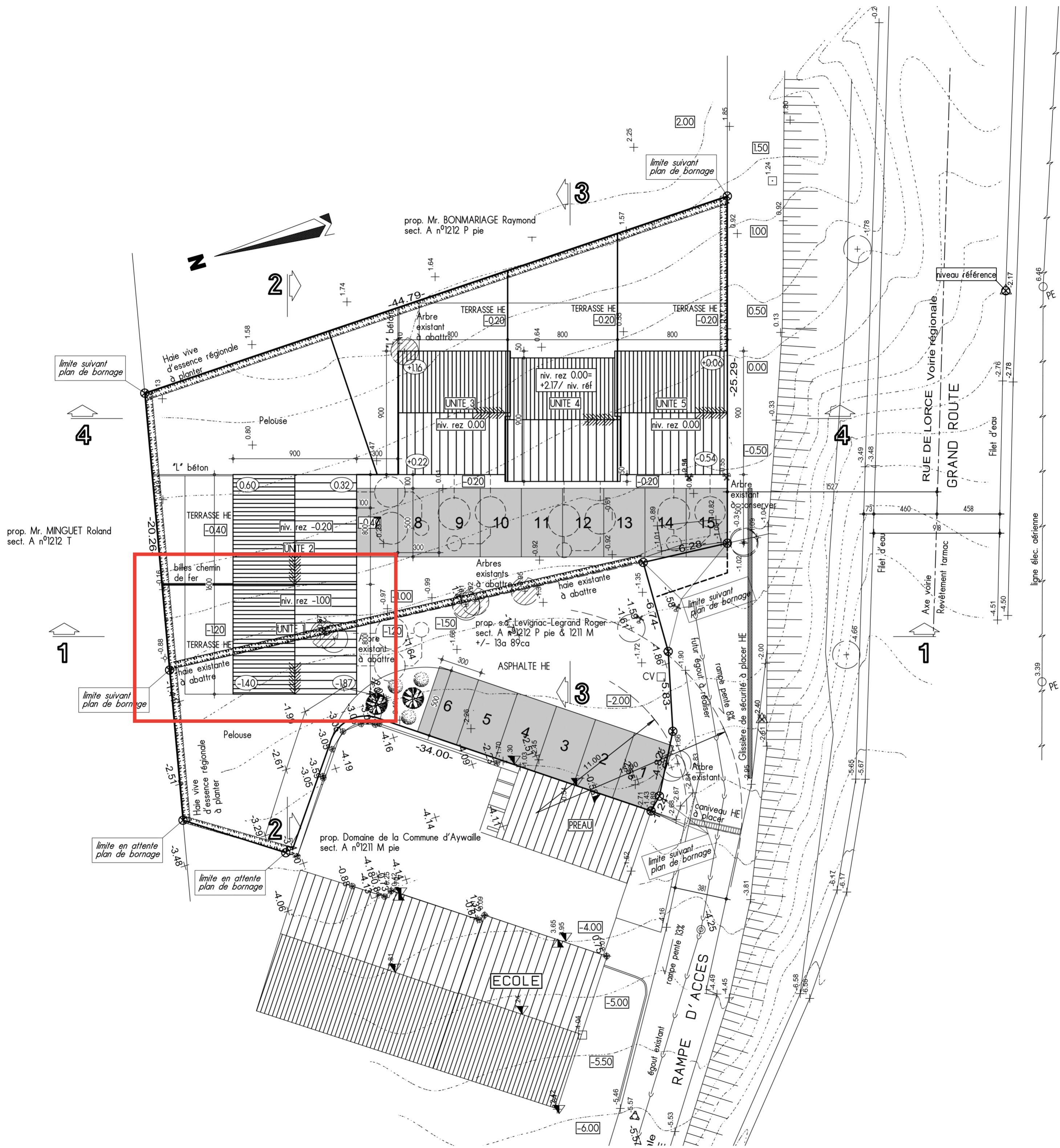
IMPLANTATION (Ech. : 1/200)
